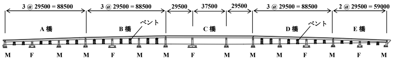
図-1 側面図
