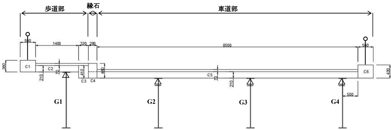
図-5 横断方向モデル
