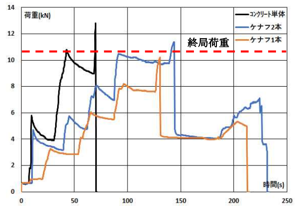
図-10 コンクリート単体、ケナフ補強 Case の载荷履歴
