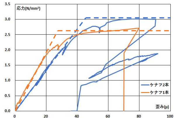
図-11 ケナフ棒の応力-歪み関係
