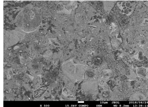
写真-4 コアAの反射電子像例
