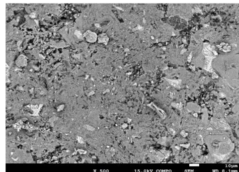
写真-6 コアJの反射電子像例
