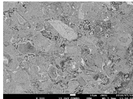
写真-5 コアCの反射電子像例
