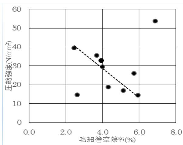
図-2 毛細管空隙率と圧縮強度
