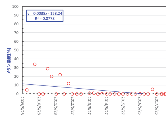
図-4 H18-9 メタンガス経年変化(減少傾向)
