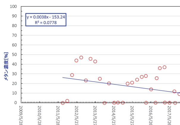
図-5 H20-2 メタンガス経年変化
