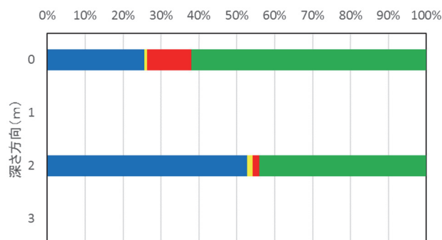
図-8 H20-2 深さガス成分分布 (2016 年 9 月)
