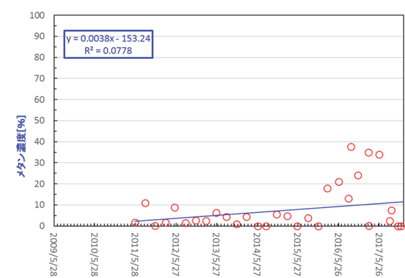
図-3 H22-6 メタンガス経年変化(増加傾向)
