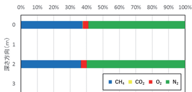
図-6 H22-6 深さガス成分分布 (2016 年 9 月)
