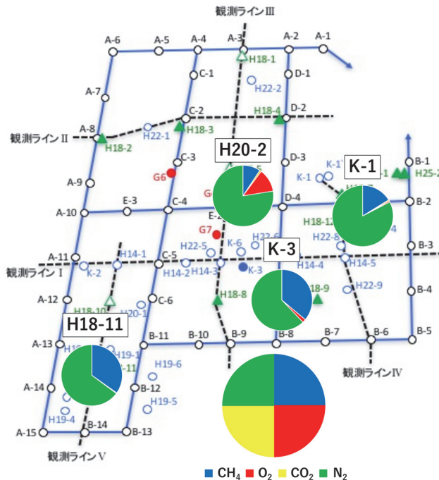
図-1 海面処分場出口ガス成分(2017年12月)
