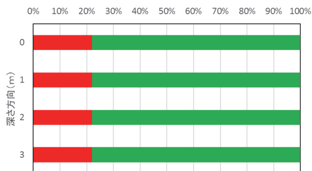
図-7 H18-9 深さガス成分分布 (2017 年 12 月)
