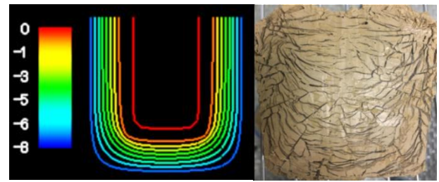
図-4.数値解析結果と断面の比較(供試体 i)
