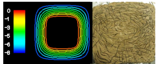
図-5.数値解析結果と断面の比較(供試体 iv)
