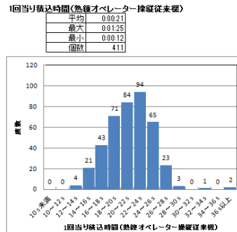
図-8 1回当りの積込み時間
