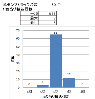
図-7 1台当り積込み回数
