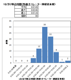
図-9 1台当たりの積込み時間
