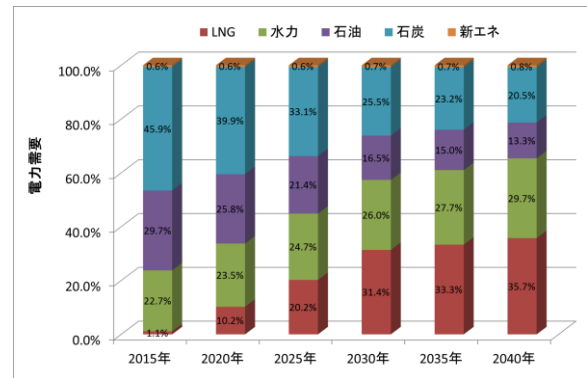
図8 原なし・火力シナリオ電力割合
