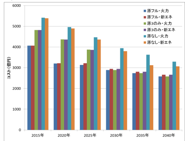
図10 発電コスト
