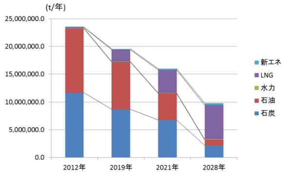
図-7 各年度の CO 2 排出量
