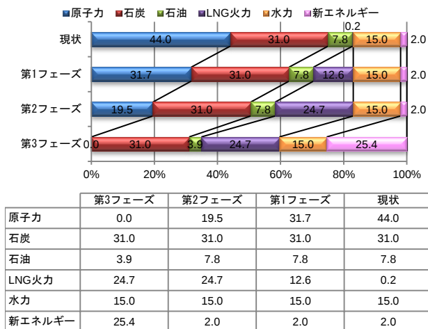
図-11 現状と脱原発後の電力構成比
