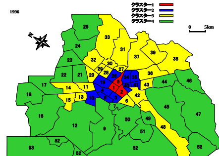
図-8 1996年のクラスター分布
