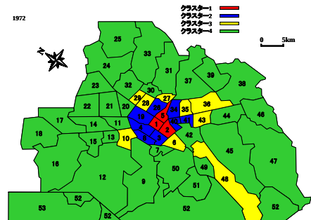
図-6 1972年のクラスター分布
