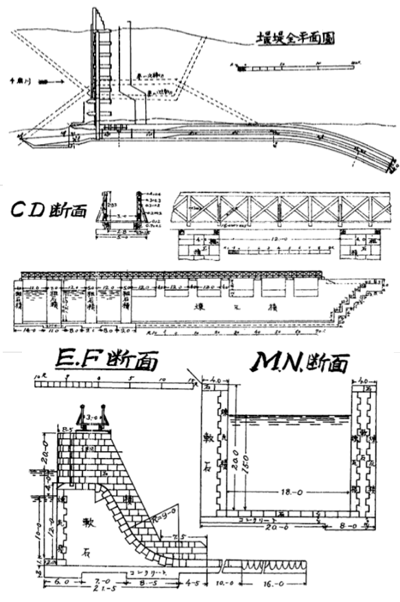
図1 千歳川第一発電所堰堤平面図および断面図 (工学会誌第337号より)
