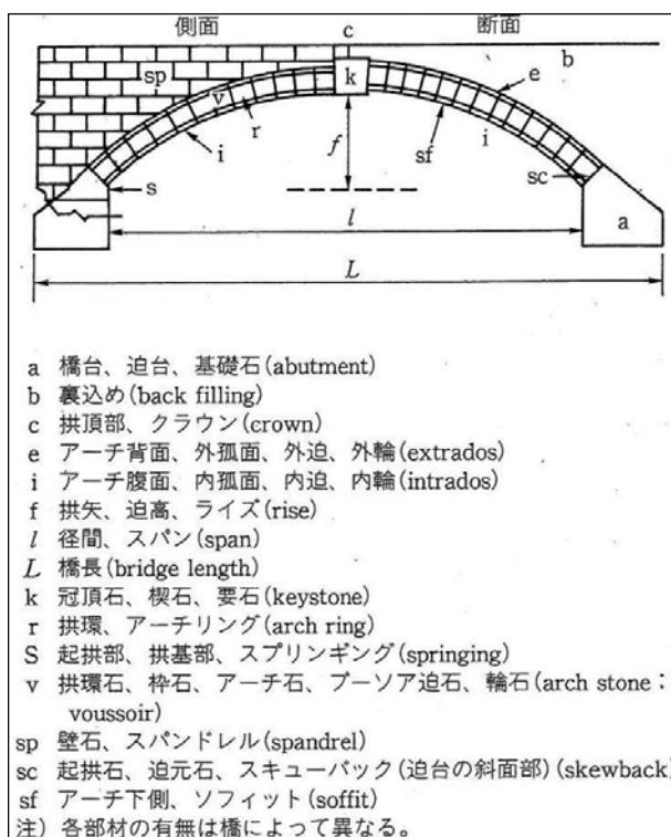
図-2 アーチ橋（拱橋）の部材名称 2)
