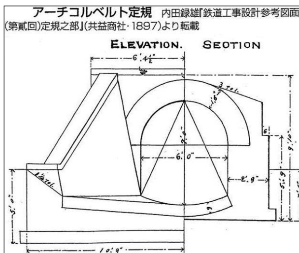
図-1 アーチコルベルト定規
