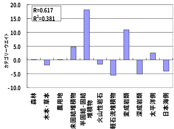
図-6 SSに対するカテゴリーウエイト
