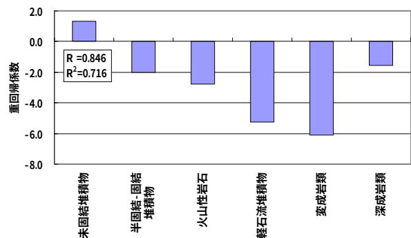
図-12 CODの地質区分別重回帰係数
