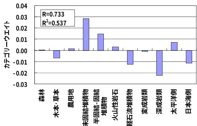
図-9 T-Pに対するカテゴリーウエイト
