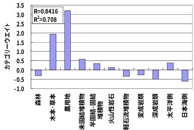
図-8 T-Nに対するカテゴリーウエイト
