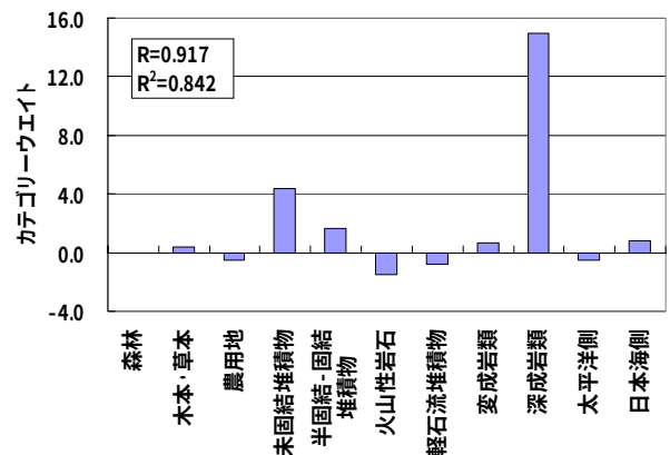
図-5 豊水・渇水流量比に対するカテゴリーウエイト 要因であるという虫明らの見解を支持する形となった。
