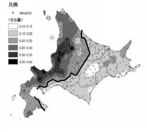
図-3 北海道の冬季降水率分布図 (太線は冬期降水率0.2の境界)
