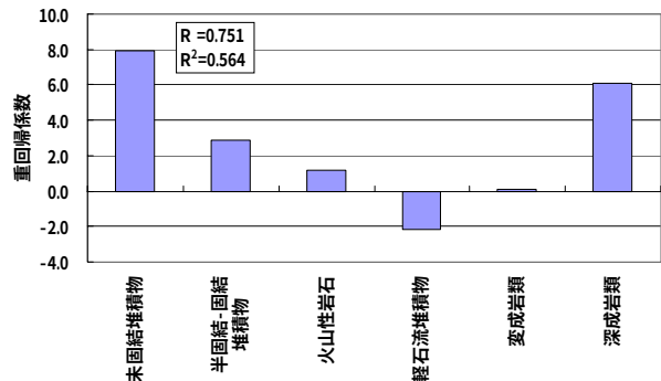
図-11 豊水渇水流量比の地質区分別重回帰係数
