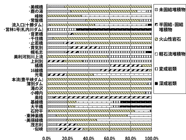
図-2 対象流域の地質
