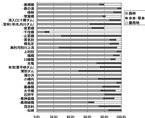
図-1 対象流域の土地利用(植生)
