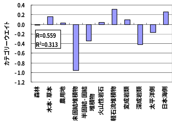
図-4 渇水比流量に対するカテゴリーウエイト
