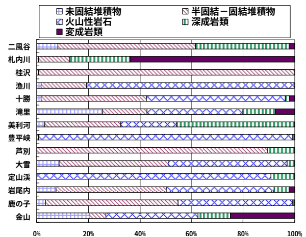
図-10 北海道のダム流域の地質面積率 10)
