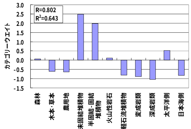
図-7 CODに対するカテゴリーウエイト
