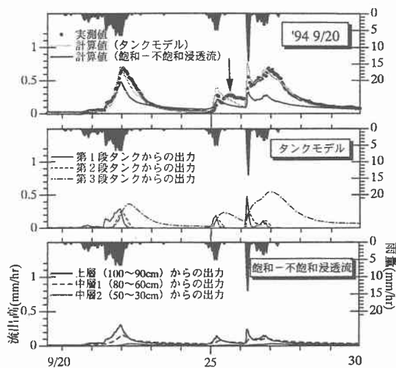
図-4 1994年9月20日の出水例と計算値
