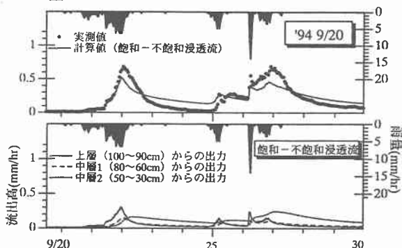
図-5 1993年10月23日の出水例と計算値
