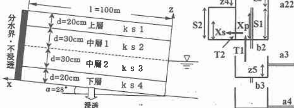
図-1 2次元断面斜面 図-2 直列4段タンクモデル
