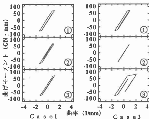
図-6(a) P2橋脚のM- \phi 関係 タイプa
