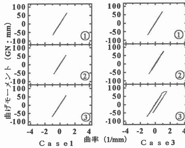
図-6(b) P2橋脚のM- \phi 関係 タイプb
