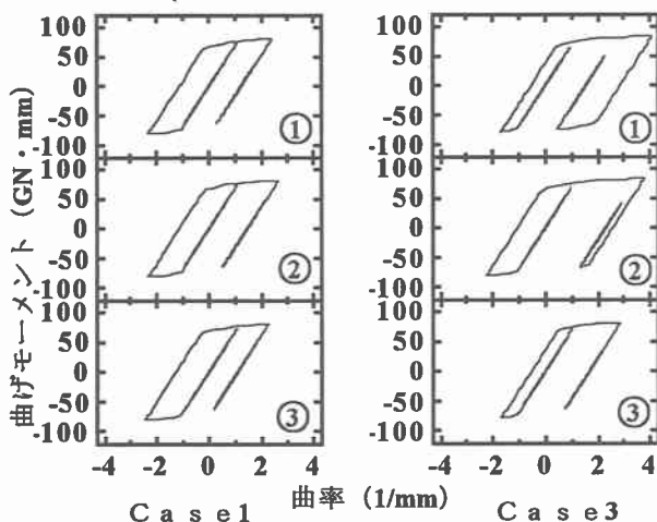
図-5(a) P1橋脚のM- \phi 関係 タイプa
