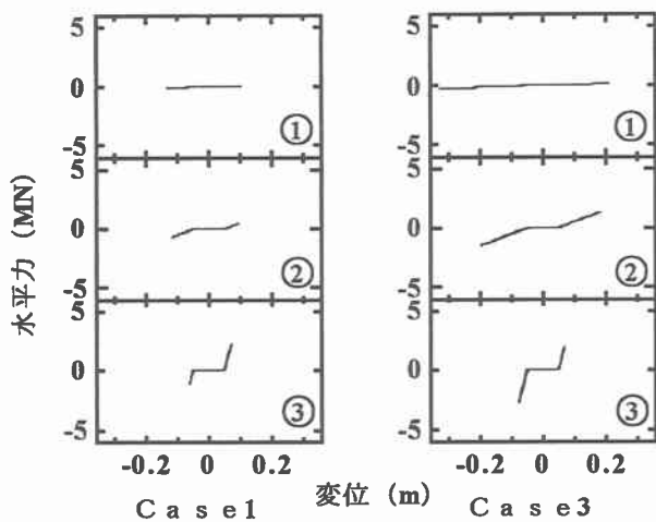
図-4(a) PC鋼棒のP- \delta 関係 タイプa
