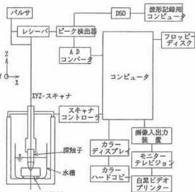
図5 測定システム
