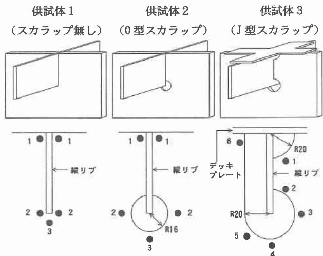
図 1 実験供試体形状と着目点
