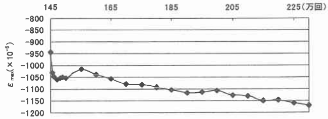
図17 着目点2のひずみ変化
