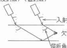
図4 直射法と1回反射法
