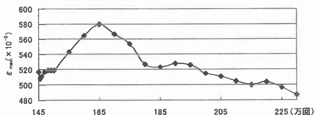
図 16 着目点 1 のひずみ変化
