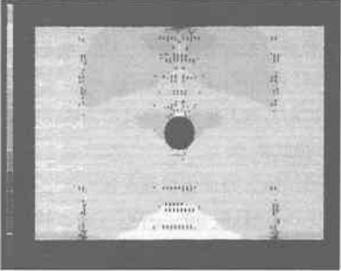
図2 水平方向応力分布
