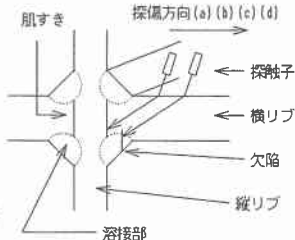
図8 超音波伝達経路 (a-a 断面)
