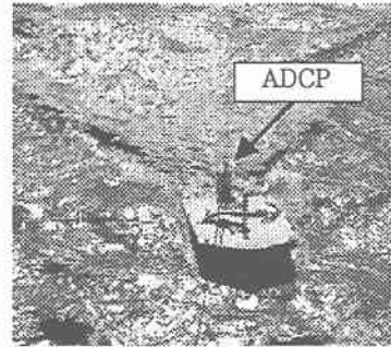
図-3 ADCP による流速測定
