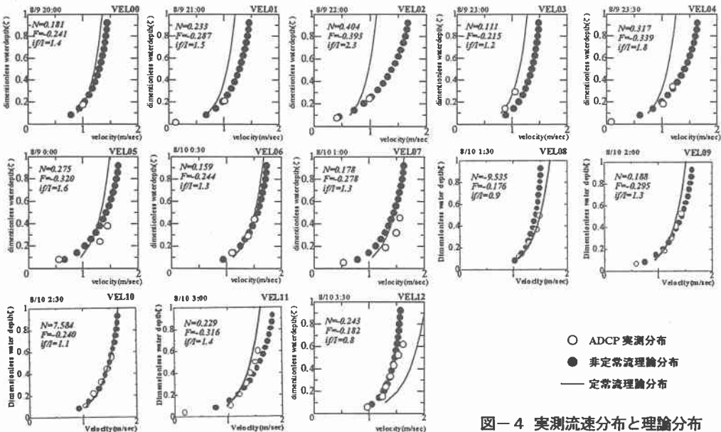
図-4 実測流速分布と理論分布
