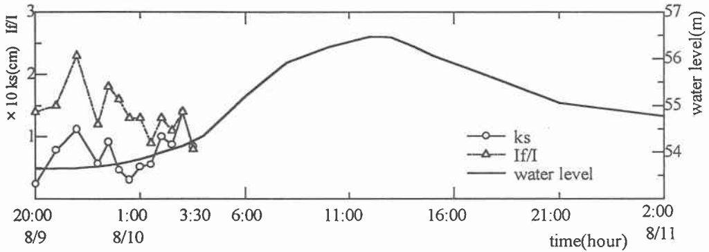
図-2 穂別橋地点のハイドログラフ
