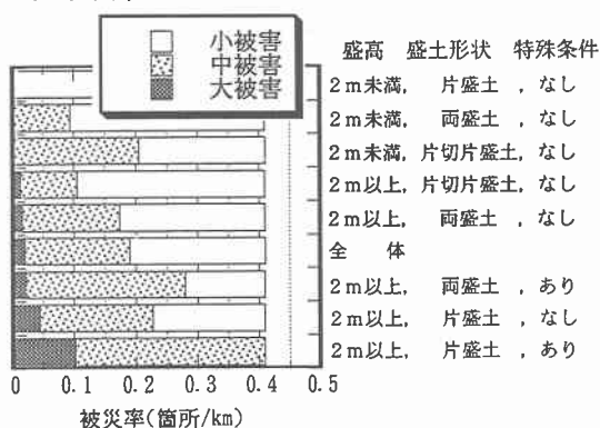
図-6 盛土条件と被災率
