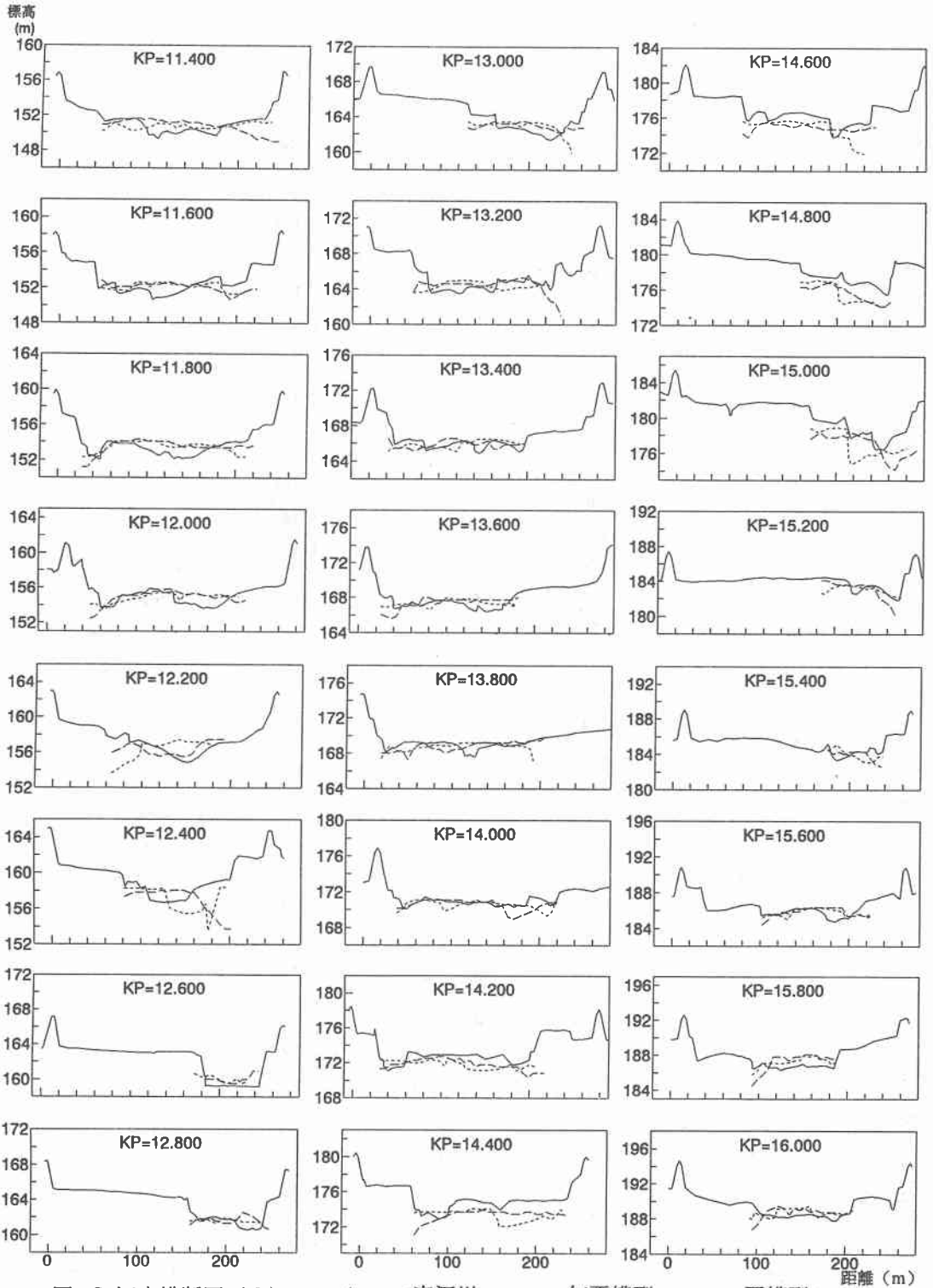
図-2 河床横断面図(2)
