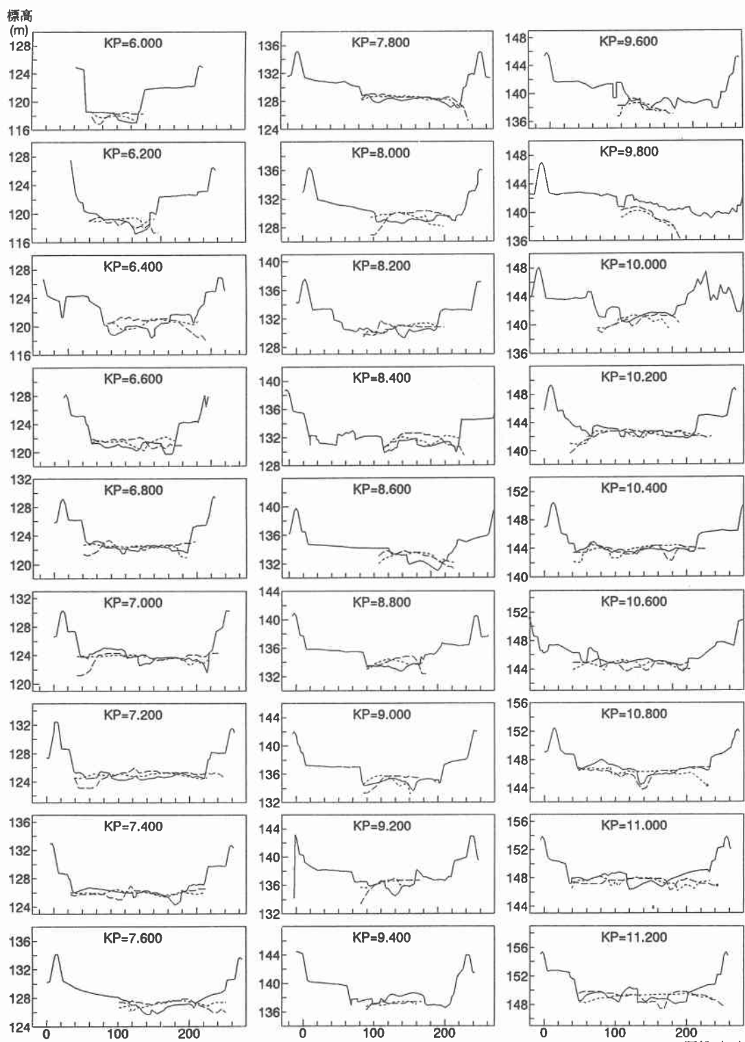
図-2 河床横断面図 (1)
