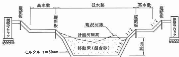
図-2 移動床模型横断形状
