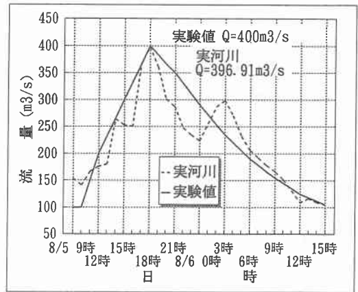
図-6 模型実験ハイドログラフ
