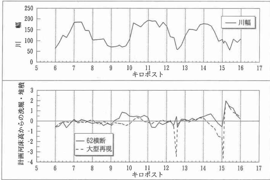
図-4 実河川と実験値の河床変動比較
