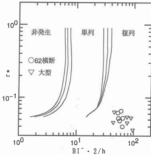
図-5 黒木・岸による砂州領域区分
