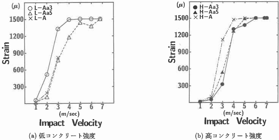
図-6 載荷速度と上部帯筋歪の関係
