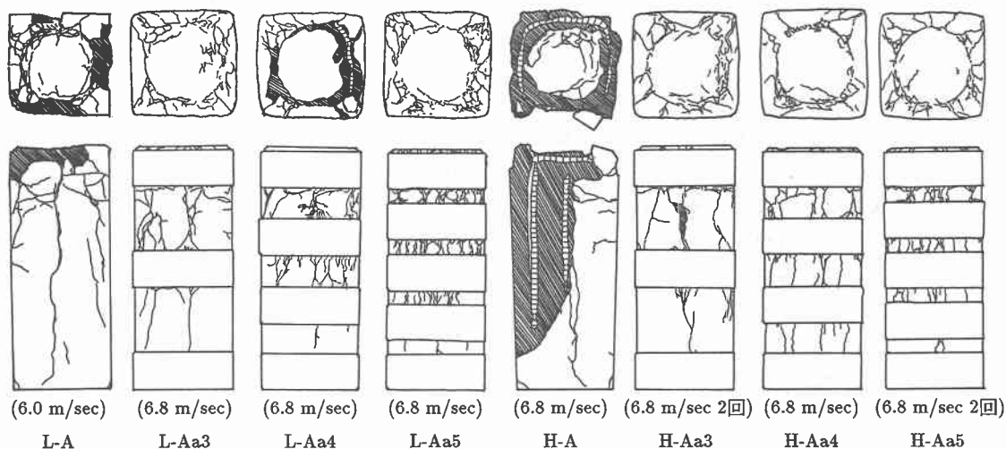
図－7 ひびわれ性状
