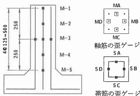
(b) 歪ゲージ取付位置
