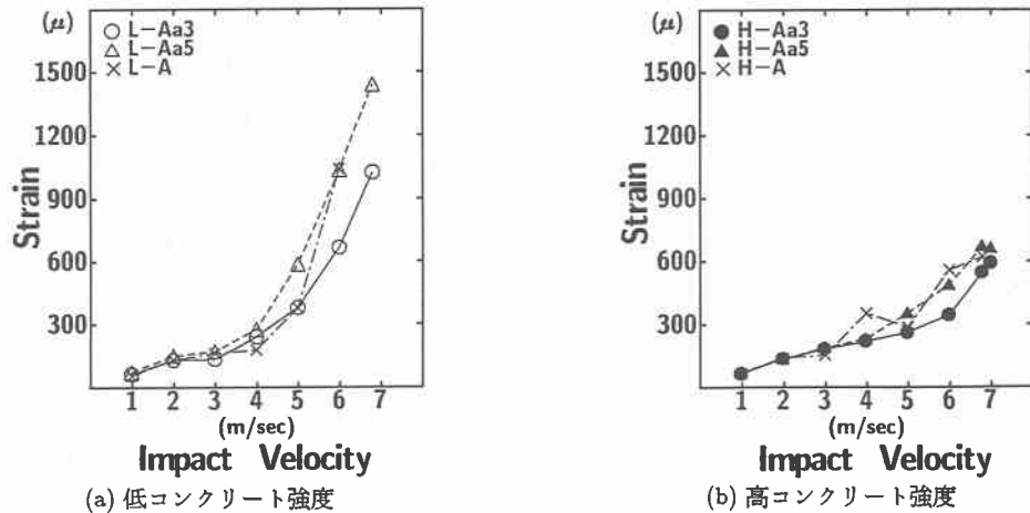
図一 3 載荷速度と軸筋中央部歪の関係
