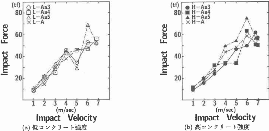
図一 2 載荷速度と重錘衝撃力の関係
