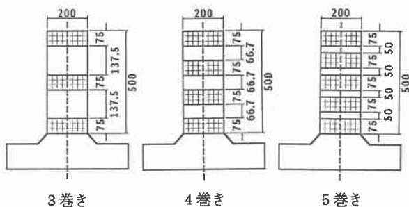
(c) アラミドテープ巻き付け位置
