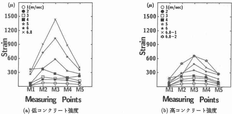
図－5 載荷速度と軸筋歪分布性状の関係 ( 5 巻き )
