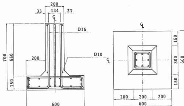
(a) 試験体形状寸法および配筋
