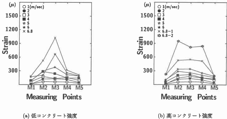
図－4 載荷速度と軸筋歪分布性状の関係 ( 3 巻き )
