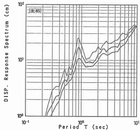
図-8 主桁での変位応答スペクトル曲線
