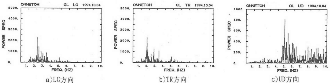
図-6 温根沼大橋のパワースペクトル
