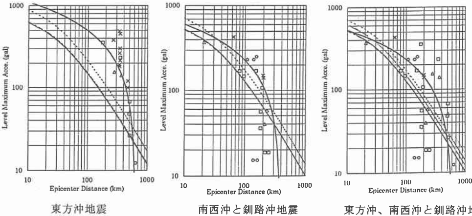
図-2 震央距離と最大加速度
