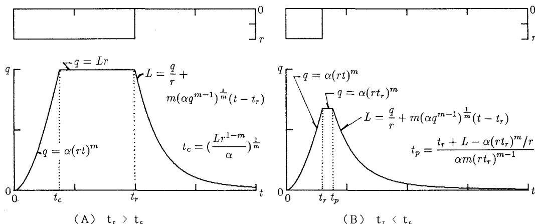
図-5 斜面末端でのハイドログラフ
