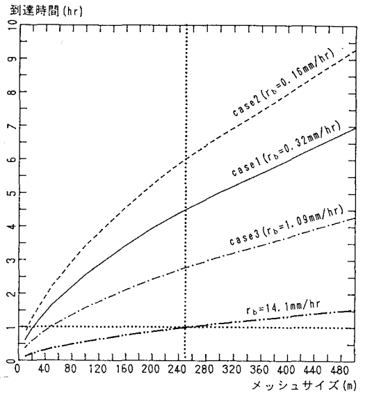
図-9 各メッシュサイズ斜面長と到達時間
