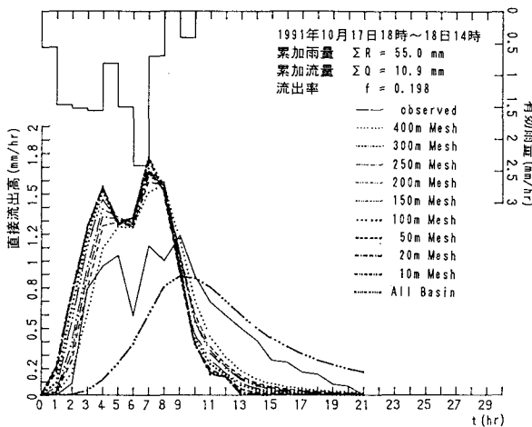
図-8 滝の沢流域における各メッシュサイズ河道網による流出計算結果と実測値との比較(case3)
