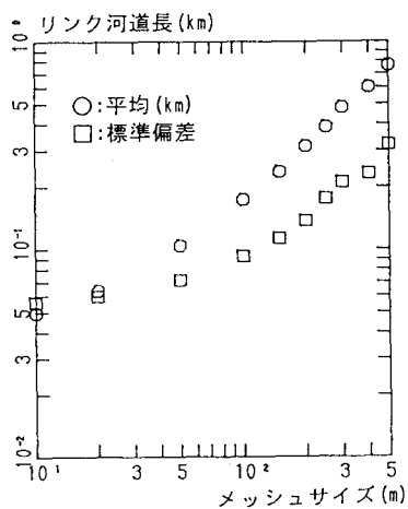
図-4(c) メッシュサイズとリンク河道長
