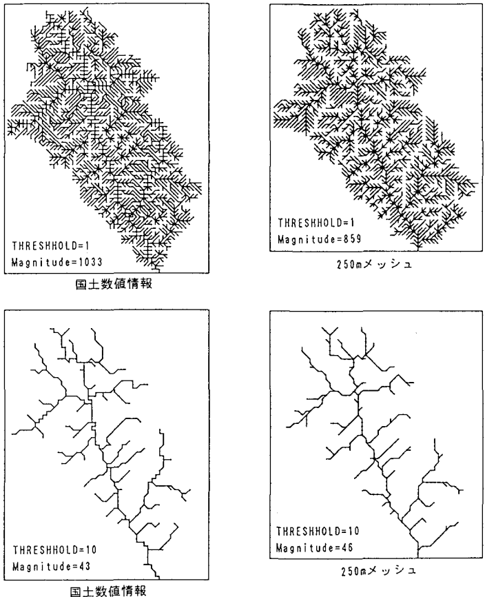
図-1 国土数値情報と10mメッシュ基準の250mメッシュ河道網比較
