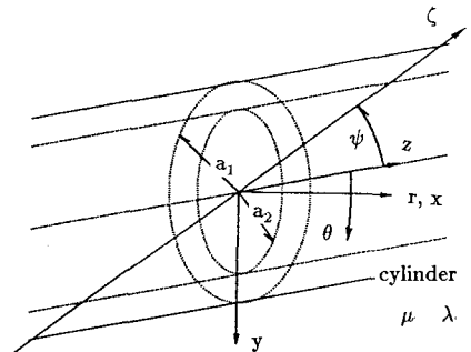
図-1 円筒座標
