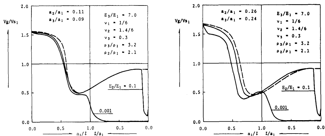
図-9 一次の軸対称波動の群速度分散曲線 (Case I)
