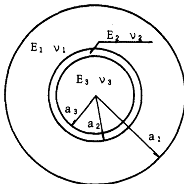
図-2 三層同心円柱
