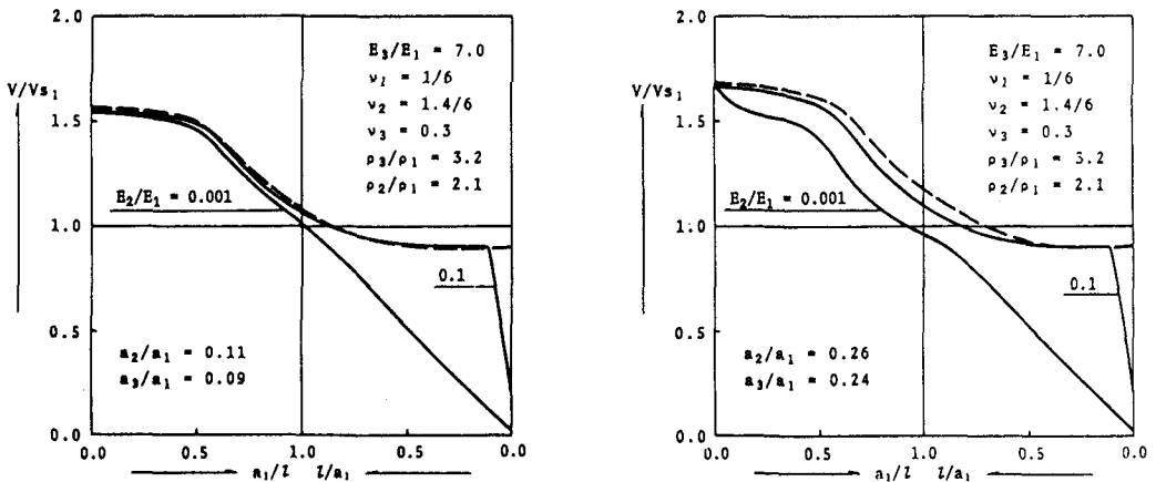
図-3 一次の軸対称波動の位相速度分散曲線 (Case I)
