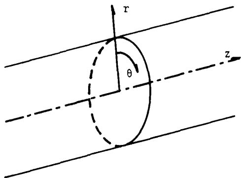
図-1 円柱座標
