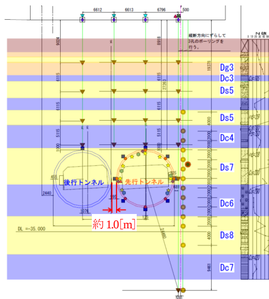
図-3 計測断面①の断面図
