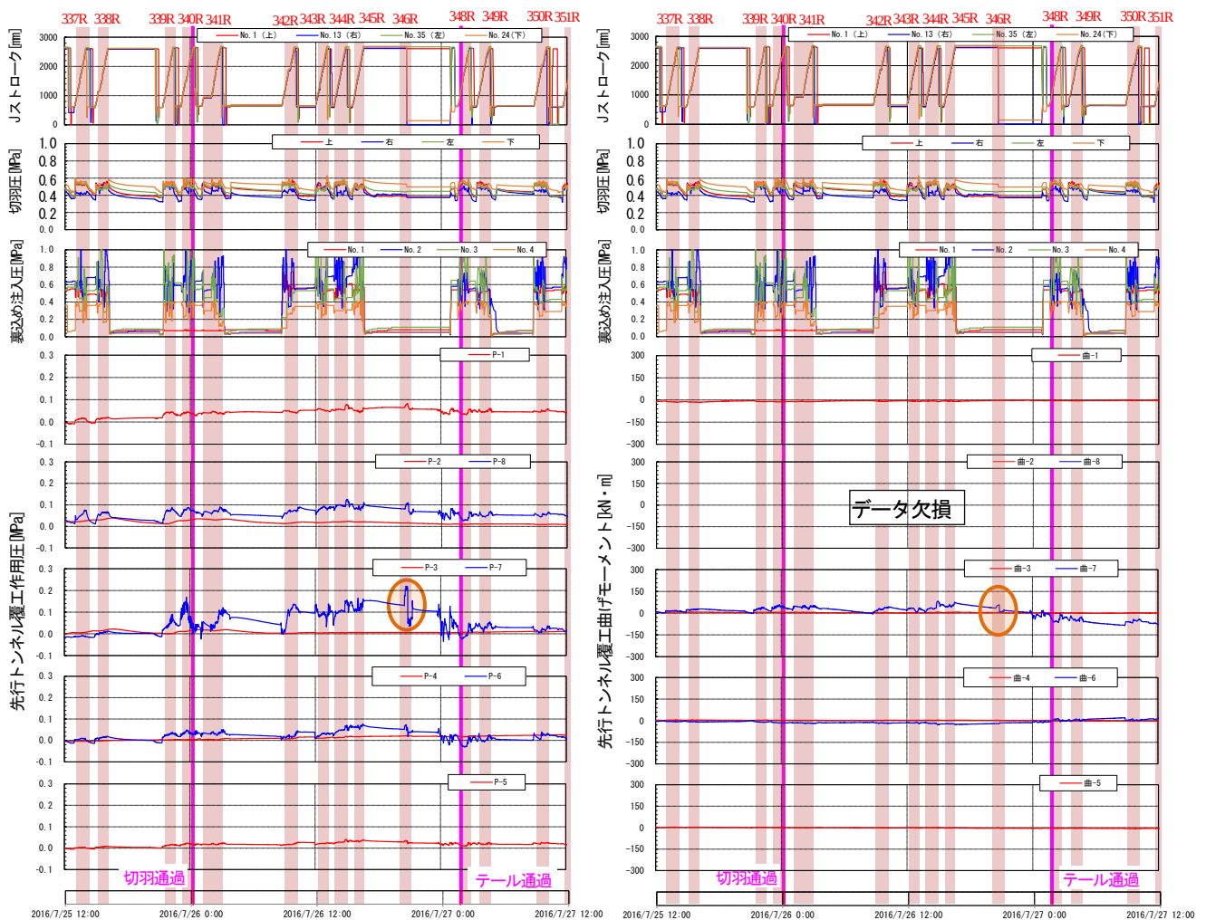
図-6 計測断面①における作用圧および曲げモーメントの経時変化図
