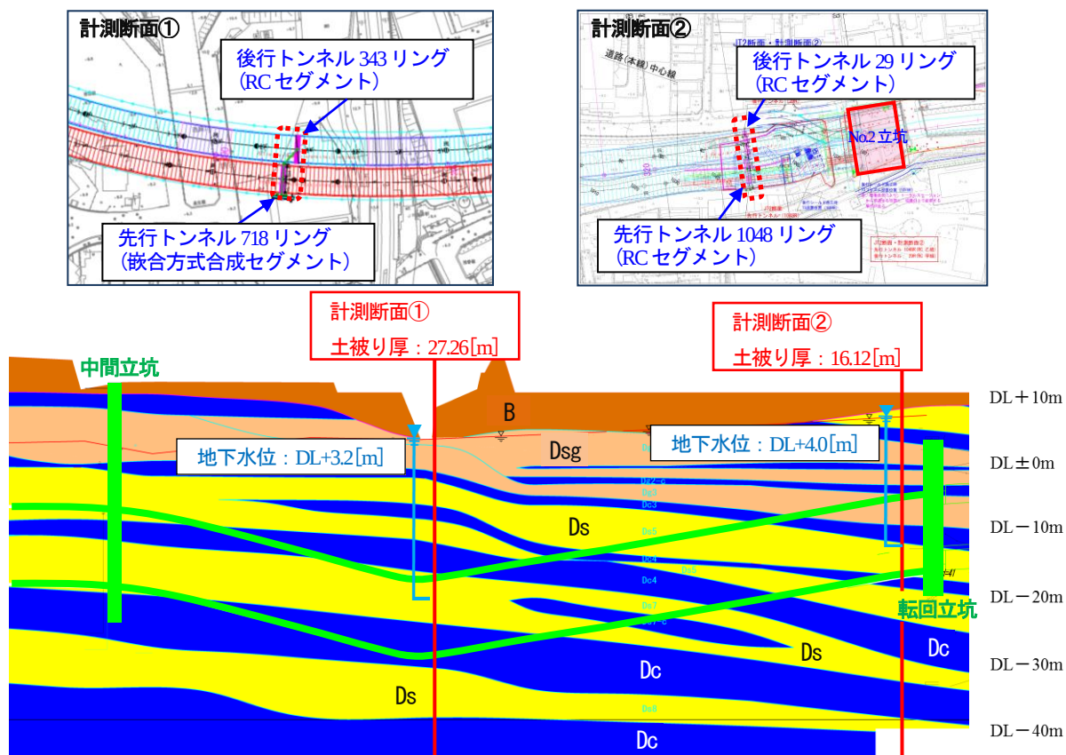
図-2 計測断面①および②の平面図および土質縦断面図
