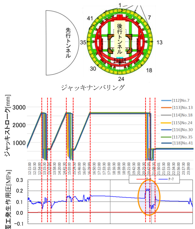
図-8 計測断面①最大作用圧発生時のマシンデータ
