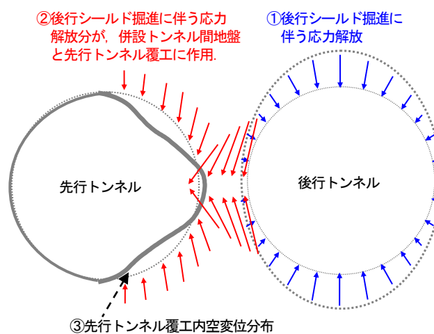
図-12 併設影響のメカニズム概念図
