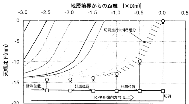
図-7 硬質層 (E=500MPa) で均質な地山のたわみ曲線
