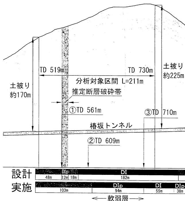
図-10 分析対象区間の地山条件と支保パターン
