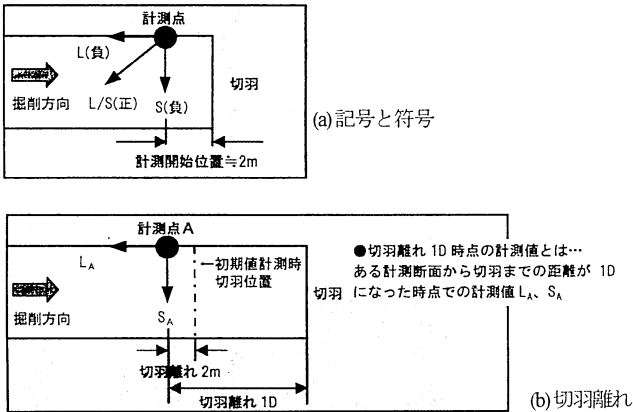
図4 切羽離れの概念図
