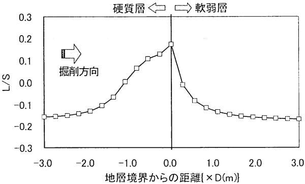
図6 馬蹄形断面モデルを用いた L/S の解析結果
