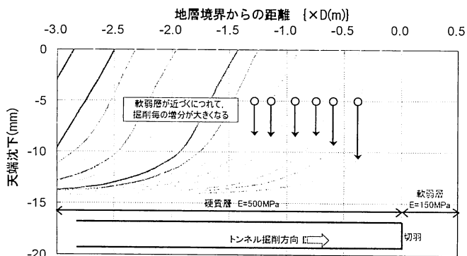
図-8 軟弱層が前方にある場合のたわみ曲線
