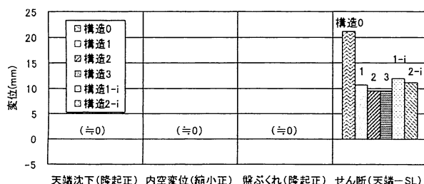
図-7 覆工構造と変位量 (せん断変形, \nu=0.30 )
