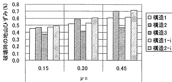
図-10 覆工破壊時の地山ひずみ (せん断変形)
