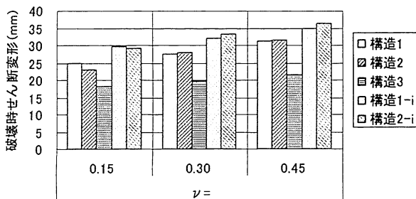
図-11 覆工破壊時の覆工変位 (せん断変形)
