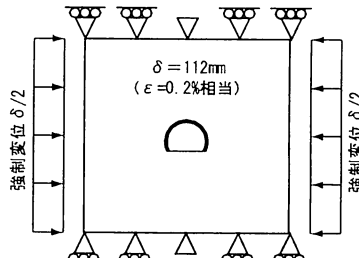
(b) 水平圧縮変形
