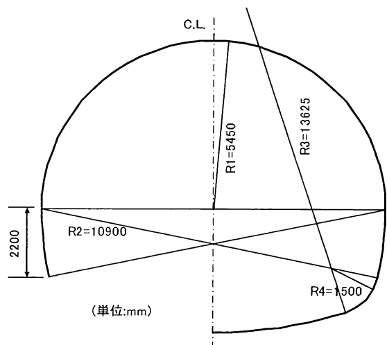
図-5 覆工（軸線）の形状寸法
