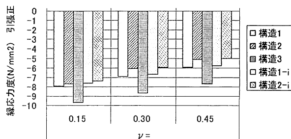
図-9 覆工肩部の圧縮応力極大値 (せん断変形)
