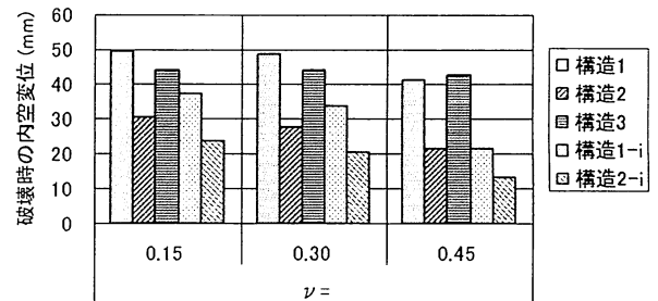
図-17 覆工破壊時の覆工変位 (水平圧縮変形)
