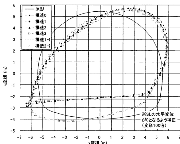
図-6 トンネルの変形モード (せん断変形, \nu=0.30 )
