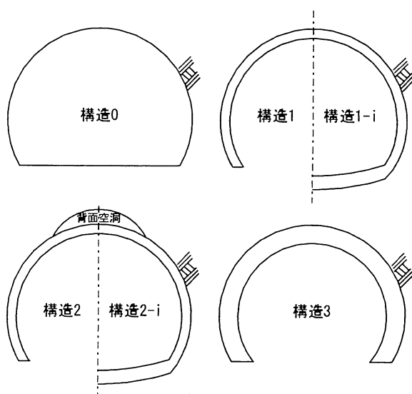
図-4 本検討で対象とした覆工構造の概念図
