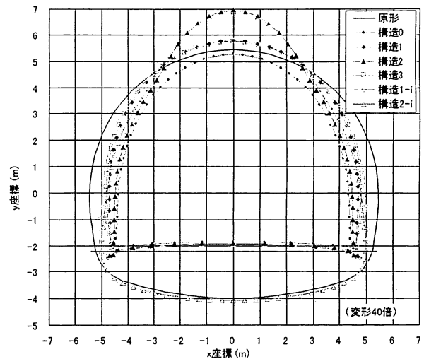
図-12 トンネルの変形モード (水平圧縮変形, \nu=0.30 )
