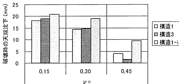
図-23 覆工破壊時の覆工変位 (鉛直圧縮変形)
