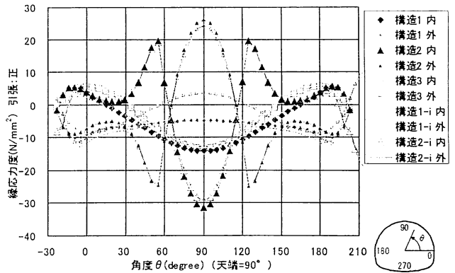
図-14 覆工の縁応力 (水平圧縮変形, \nu=0.30 )
