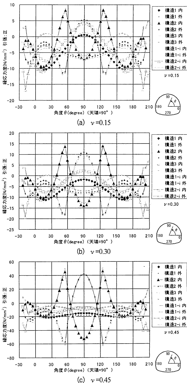
図-20 覆工の縁応力 (鉛直圧縮変形)
