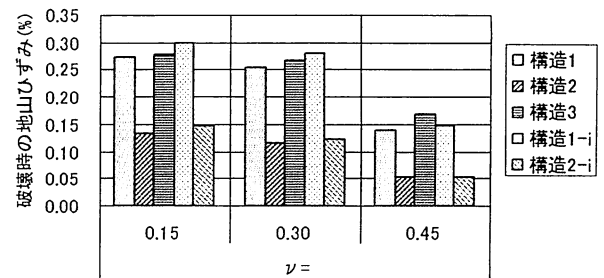
図-16 覆工破壊時の地山ひずみ (水平圧縮変形)
