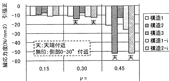
図-21 覆工の圧縮応力極大値 (鉛直圧縮変形)
