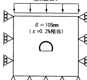
(c) 鉛直圧縮変形
