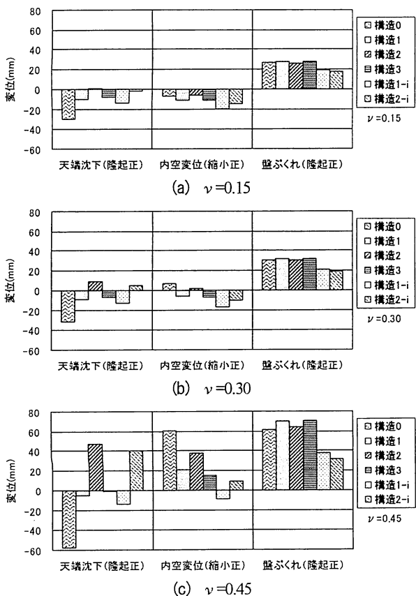
図-19 覆工構造と変位量 (鉛直圧縮変形)
