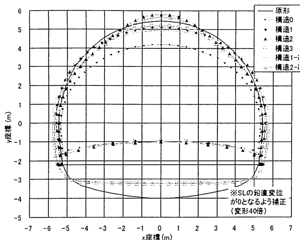
図-18 トンネルの変形モード (鉛直圧縮変形, \nu=0.30 )
