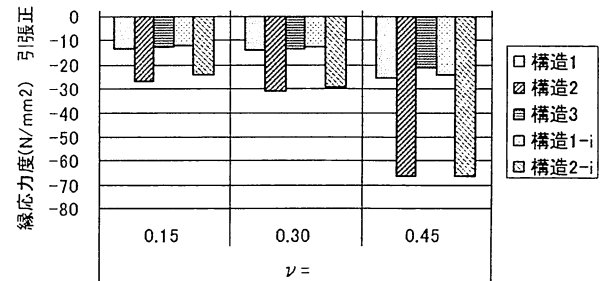
図-15 覆工天端の圧縮応力極大値 (水平圧縮変形)
