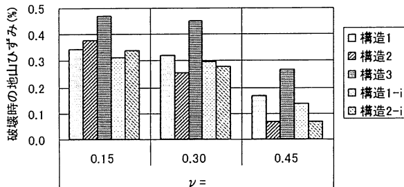
図-22 覆工破壊時の地山ひずみ (鉛直圧縮変形)
