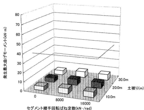
図-5 良質地盤（正曲げ）
