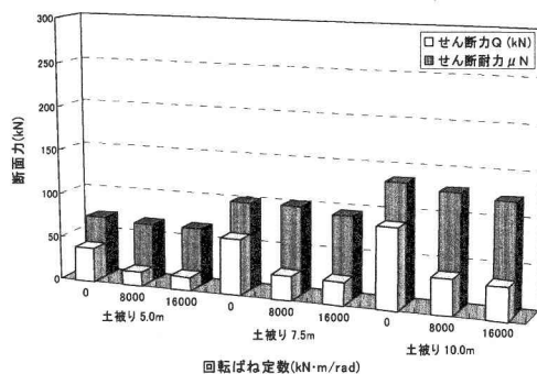
図-8 せん断照査結果（軟弱地盤）
