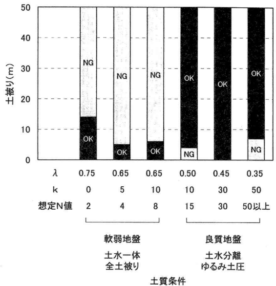
図-18 土質条件による適用範囲
