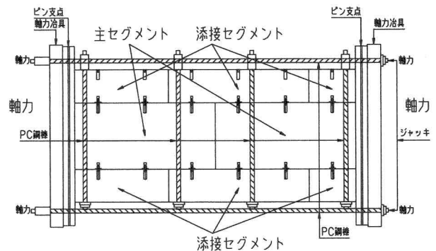
図-12 添接曲げ試験方法
