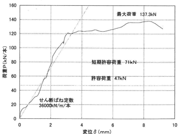
図-17 せん断荷重ー変位図
