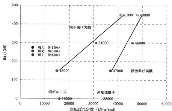
図-14 軸力ー回転ばね定数相関図
