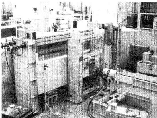
図-11 継手曲げ試験状況
