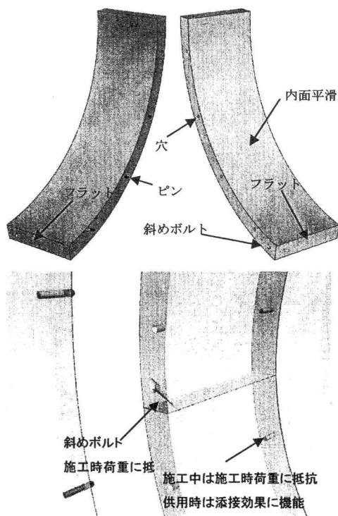
図-1 セグメント構造概要図
