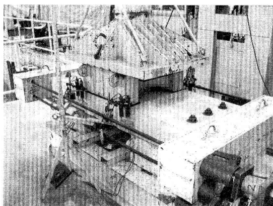
図-16 リング間せん断試験状況
