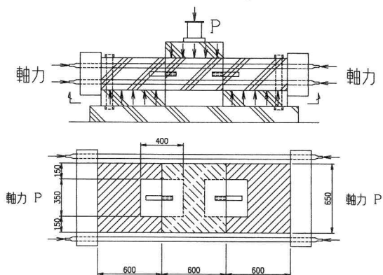
図-15 リング間せん断試験方法
