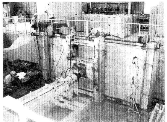
図-13 添接曲げ試験状況
