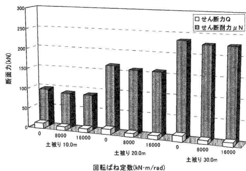
図-9 せん断照査結果（良質地場）
