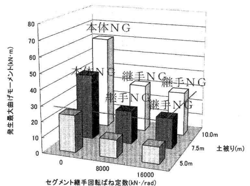
図-3 軟弱地盤 (正曲げ)
