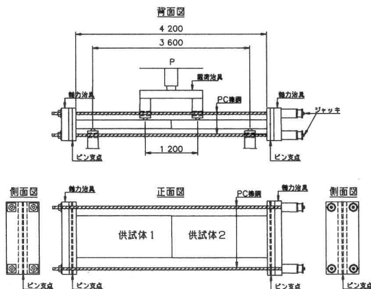
図-10 継手曲げ試験方法
