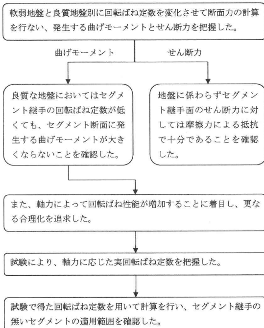
図-2 適用性検討フロー図
