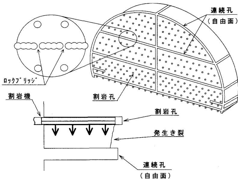
図-1 割岩工法概念図
