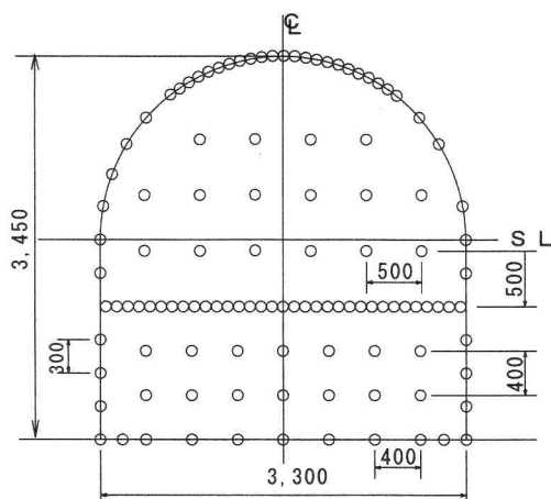
図－8 B避難連絡坑における穿孔パターン
