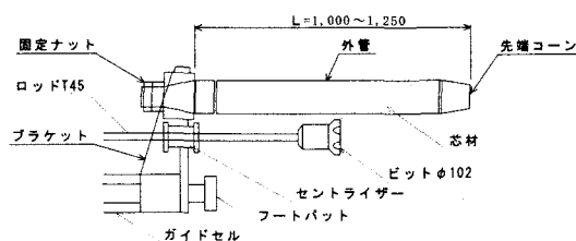
図-2 SABロッド装着状況
