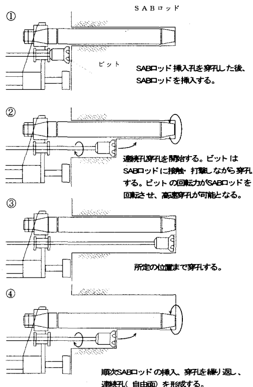
図-3 連続孔穿孔手順
