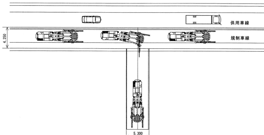
図－４ A 避難連絡坑における削岩機の機械配置
