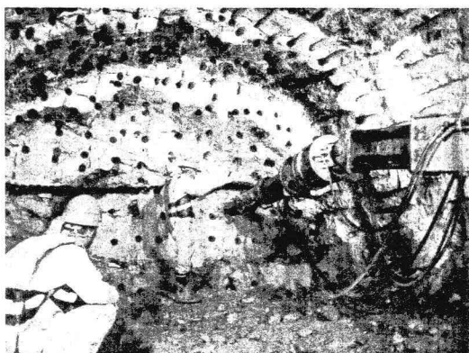
写真－1 A避難連絡坑における割岩状況
