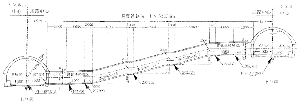
図-7 B避難連絡坑縦断面図
