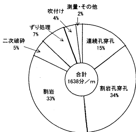
図-6 A避難連絡坑におけるサイクルタイムの一例
