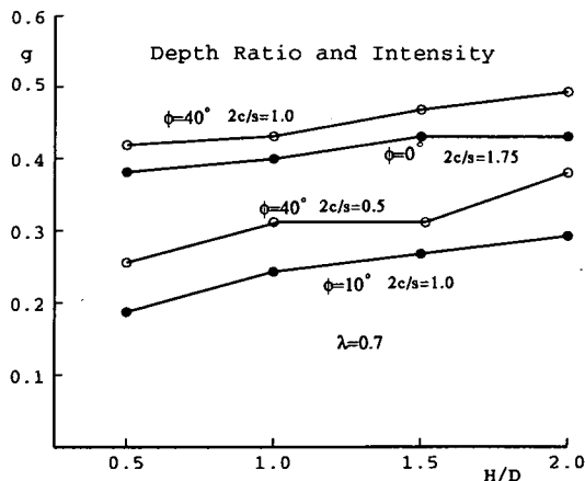
図 3: 土被り比と限界震度の関係
