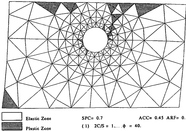
図 1: 解析結果の一例 ( H/D=1.0 )
