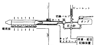
図-7 孔内載荷試験
