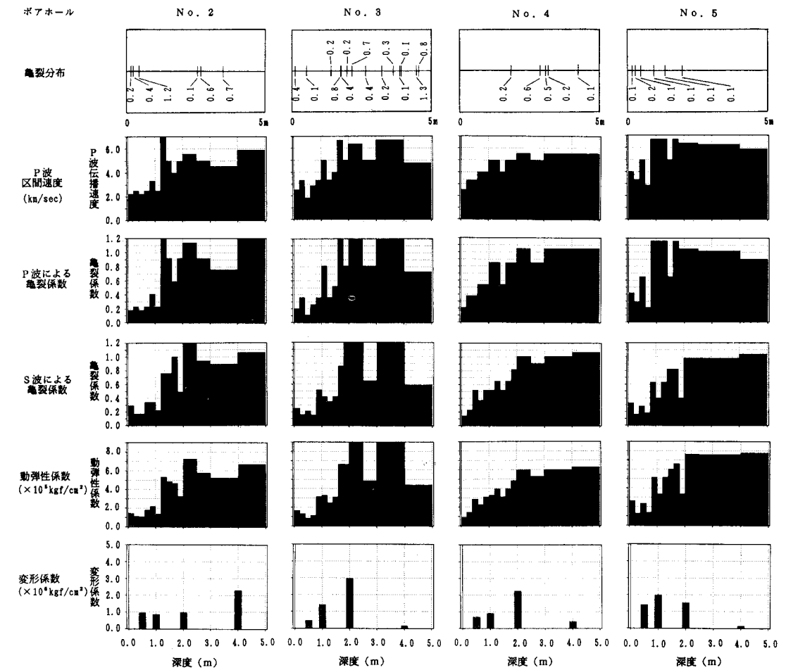
図-10 No. 2～No. 5 ボアホールの調査結果
