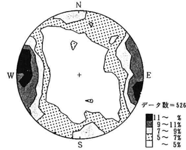
図-2 亀裂分布図 (ウルフネット下半球投影)
