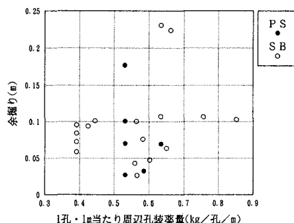
図-8 周辺孔装薬量と余掘りの関係
