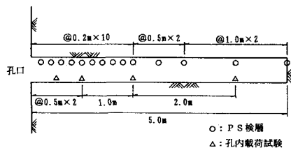
発破パターンが異なる場所における発破の影響度の違いを調べるために、4ヶ所において掘削後トンネル軸に対して垂直な方向に孔長5mのボーリング孔（口径76mm、仰角10°）を設け、それぞれのボアホールにおいて各種孔内試験を実施した。
