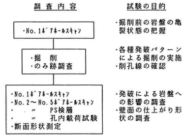
図-3 調査試験フロー
