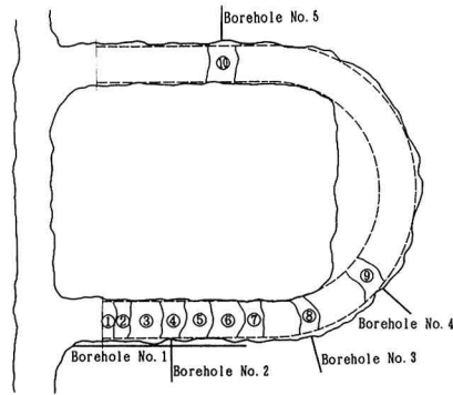
図-4 試験場平面図
