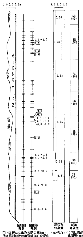
図-9 掘削前後の亀裂変化
