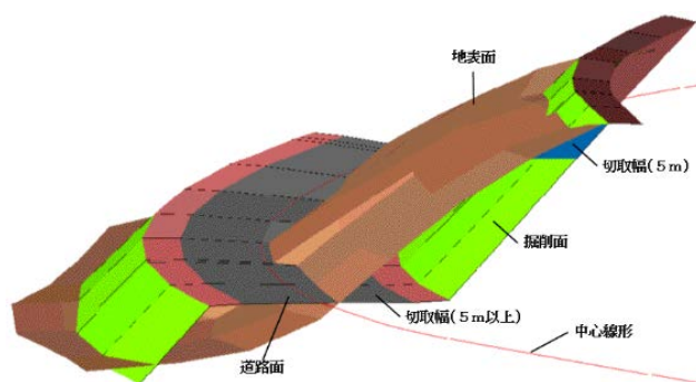
図-2 土工モデル
