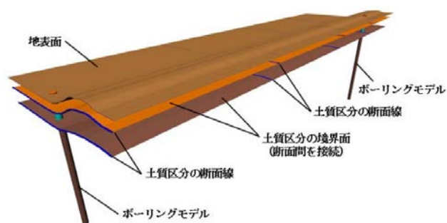
図-1 3次元地盤モデル
