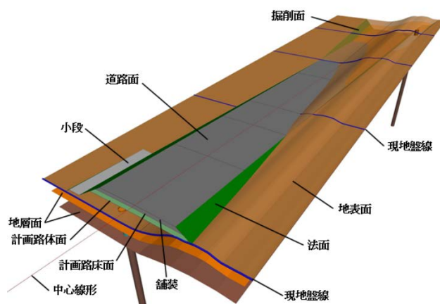
図-3 土構造物の3次元モデルの例
