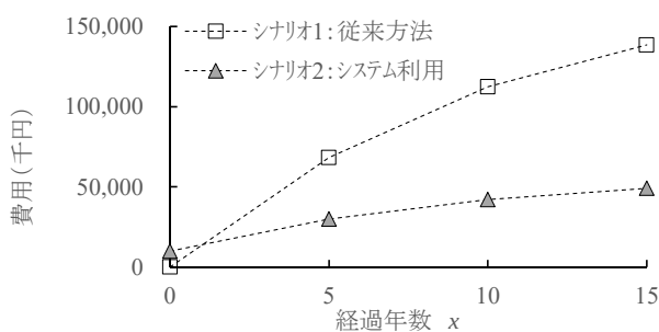
図-7 提案するシステム導入による経済効果例
