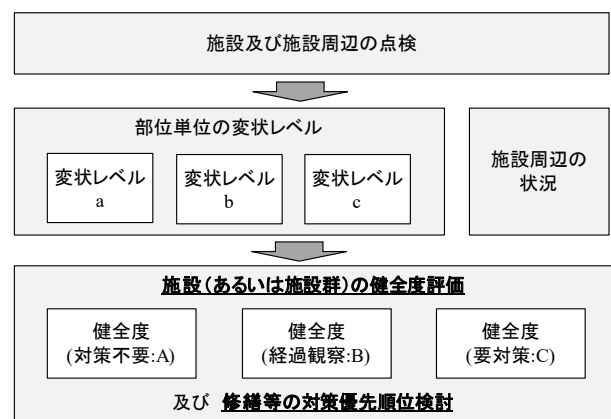
図-1 砂防関係施設の維持管理（長寿命化）計画の流れ 7)
