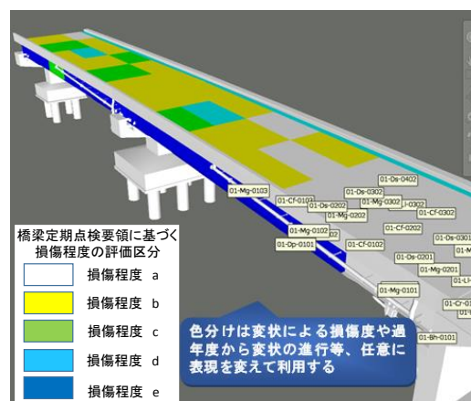
図-4 変状箇所や損傷箇所の俯瞰的な表現
