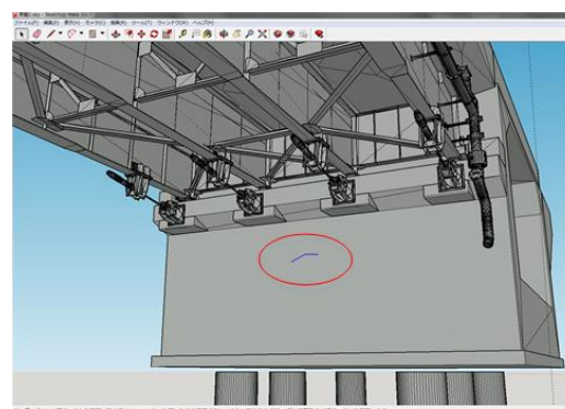
図-5 3次元的な損傷位置の記録
