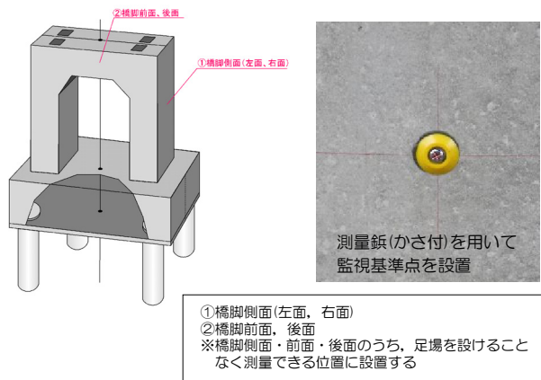
図－２ 監視基準点設置位置および設置状況例
