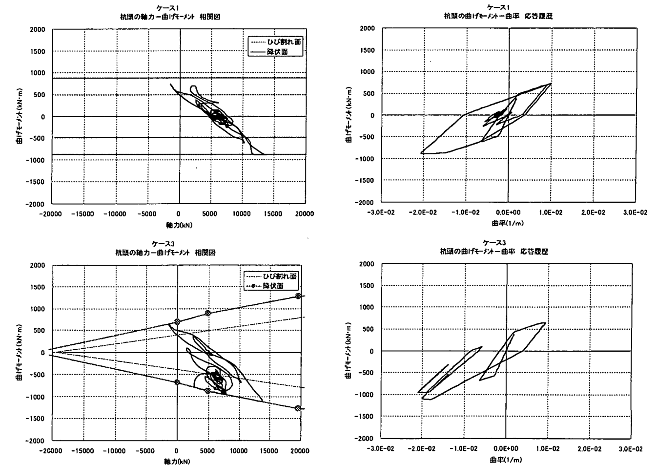
図 6 解析条件の違いによる杭頭の軸力と曲げモーメントの相関関係および曲げモーメントと曲率の関係
