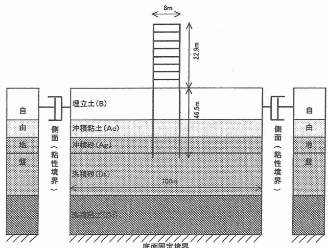
図1 解析モデル
