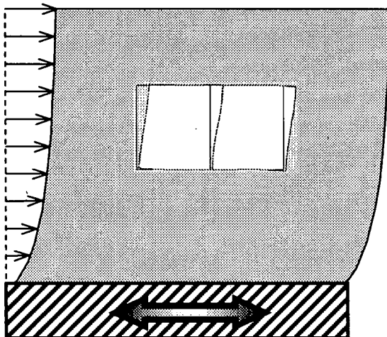
図-1 地中構造物横断方向の耐震設計
