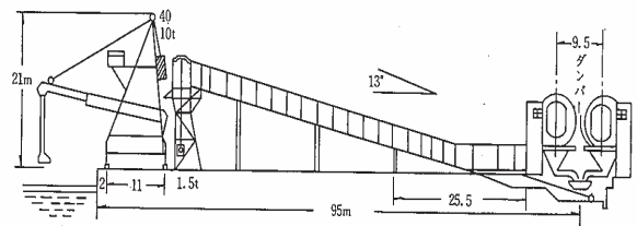
図-3 ローダー (石炭積み込み機) (文献 10,p45)
