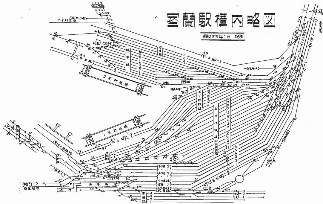
図-5 室蘭駅構内配線略図 (1964 (昭和 39) 年 1 月) (文献 10, p96)
