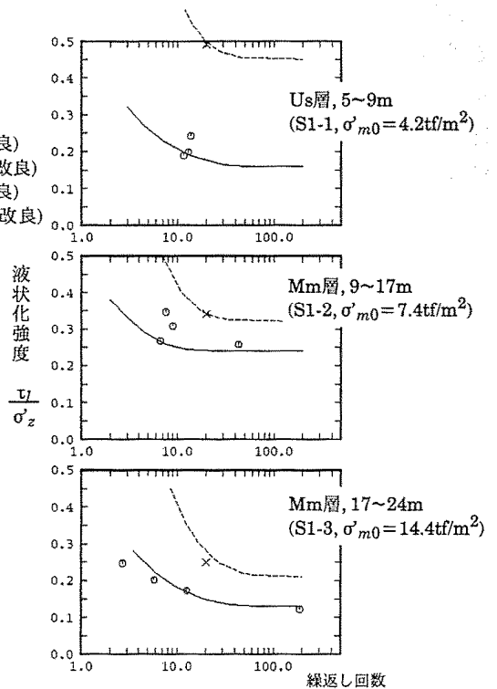
図7 液状化強度曲線 (非排水繰返し強度～繰返し回数) (移設地)
