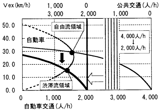
図 1 5 総需要減で渋滞発生
