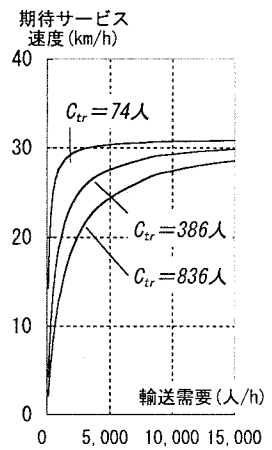
図7 編成定員 C_{tr} の影響
