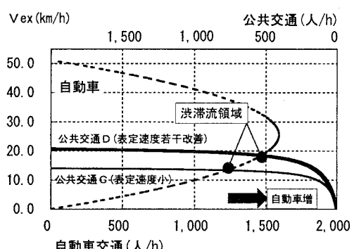
図11 公共交通の小規模な水準向上で乗客減
