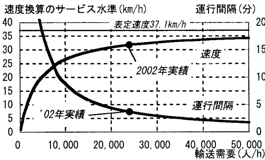
図2 輸送需要と運行間隔・速度の関係
