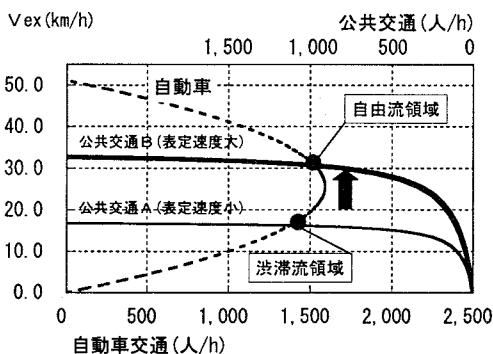
図10 公共交通の水準向上で渋滞解消
