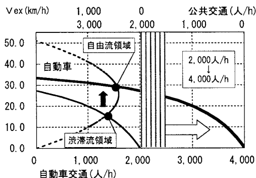
図 1 4 総需要増でも車線増設不要+渋滞解消
