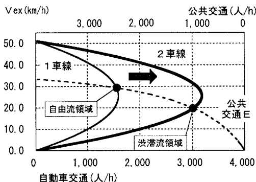
図 1 2 車線増設で渋滞発生
