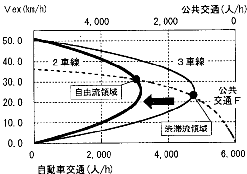
図 1 3 車線削減と良質な公共交通で渋滞解消
