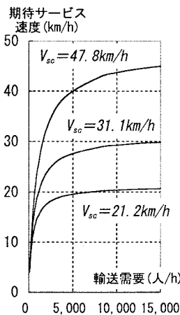
図5 表定速度 V_{sc} の影響
