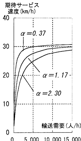
図6 混雑率 \alpha の影響
