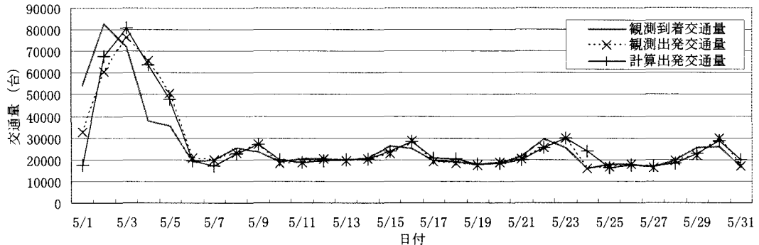
図2 交通量分布発生法による計算値と実測値のプロット (1年目1ヶ月)
