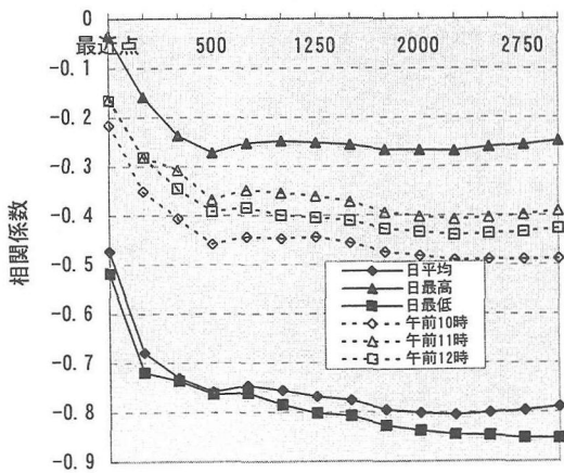
図—1 NVI採取範囲と相関係数(1992.4.21)
