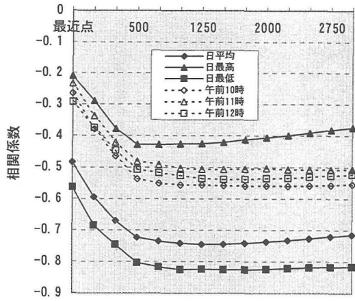
図—3 NVI採取範囲と相関係数(1987.6.27)
