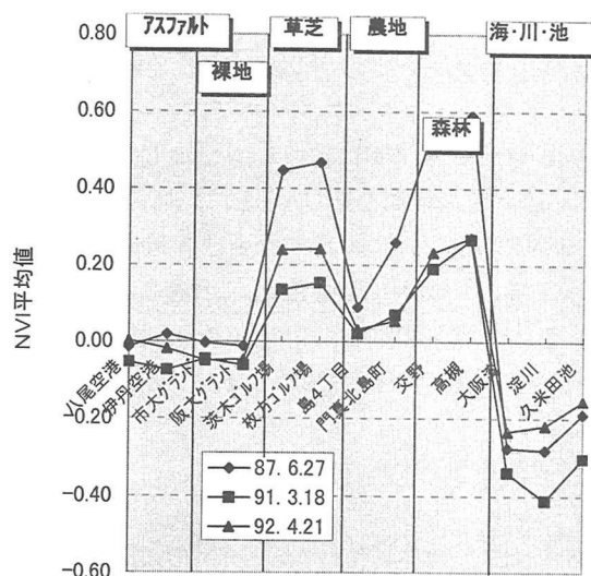
図-5 地表面被覆とNVI
