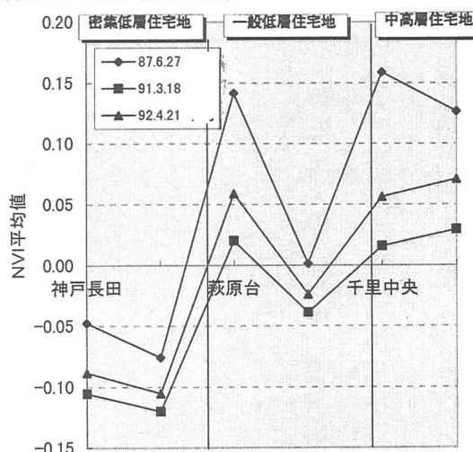
図-6 各住宅地区のNVIの平均
