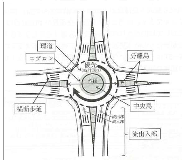
図-1 ラウンドアバウト標準図 9)
