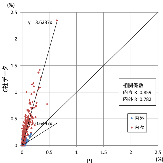
図-10 C社データとの小ゾーンOD量 (割合) の比較
