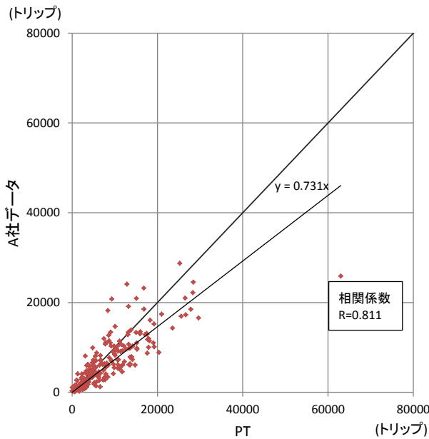
図-2 A社データとの小ゾーン集中量の比較
