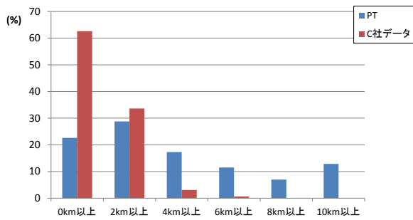
図-9 C社データとのトリップ長分布の比較
