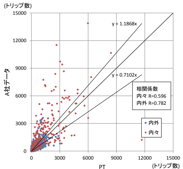
図-4 A社データとの小ゾーンOD量の比較
