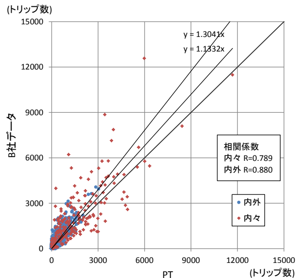
図-7 B社データとの小ゾーンOD量の比較
