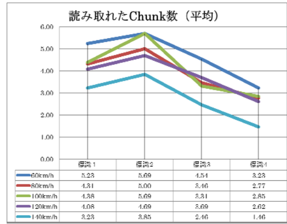
図-8 各地点で読み取れた chunk 数 (平均値)
