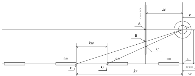
図-1 高速道路前方映像CGモデル（立面図）
