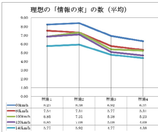
図-12 各地点での理想的な chunk 数 (平均値)
