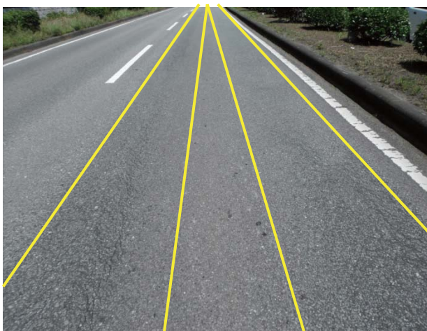
図-3 旭地区のわだち掘れ箇所状況
