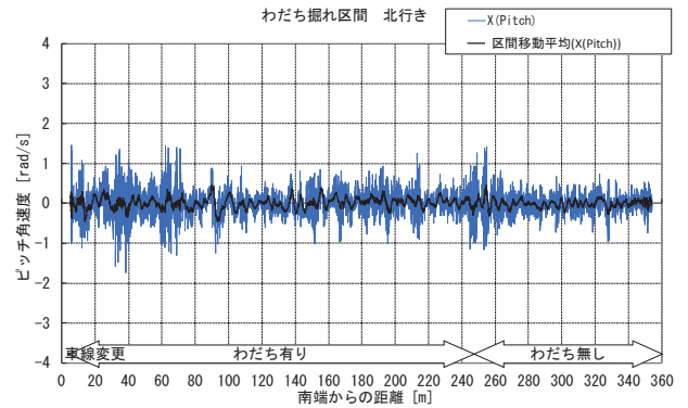
図-26 わだち掘れ区間ピッチ角速度 (北行き)
