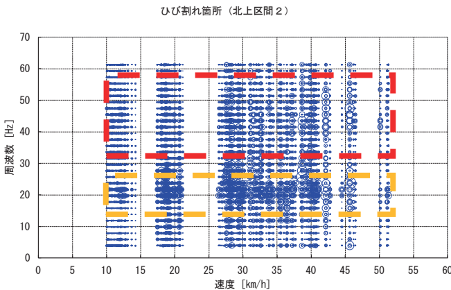
図-24 ひび割れ区間周波数スペクトル(南行き)
