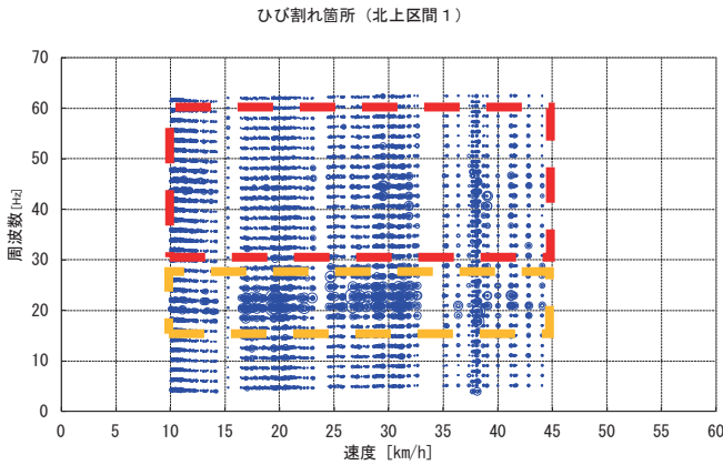
図-23 ひび割れ区間周波数スペクトル(南行き)
