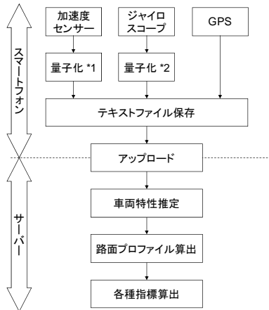
図-7 センサーデータの計算フロー
