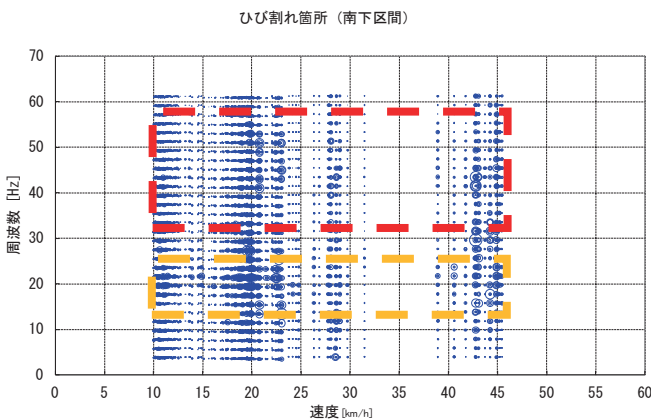
図-25 ひび割れ区間周波数スペクトル(南行き)
