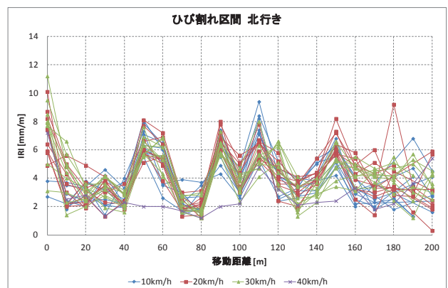
図-12 ひび割れ区間IRI (北行き)
