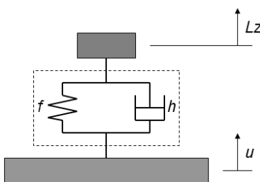
図-8 1 質点系バネモデル
