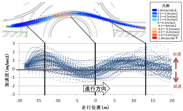
図-7 走行位置と加速度変化 (n=93)
