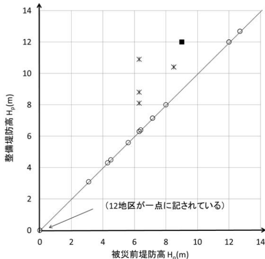
図1において整備堤防高 H_p が算出堤防高 H_c を下回った集団についてプロット ■: 田野畑村明戸海岸 *: 各海岸毎の再津波シミュレーションが行われ、その結果に余裕高1mを加えた堤防高を選択した海岸。(陸前高田市内の18か所中の6か所) ○: その他の海岸地域
